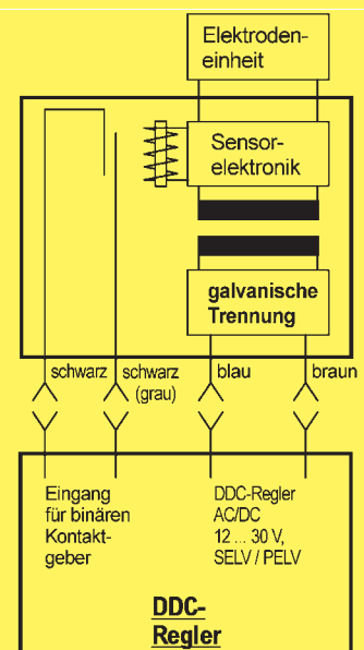
Folgeschaltung
