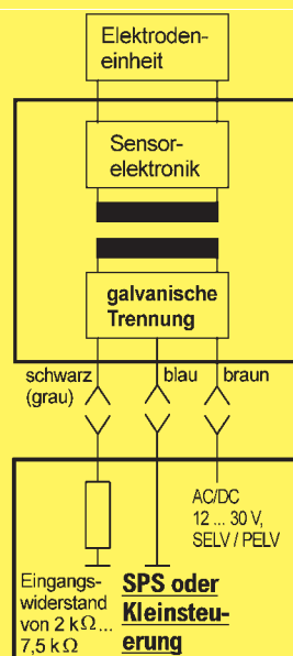
Folgeschaltung
