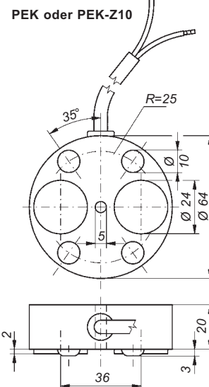
PEK-Z10, Anschlussseite
