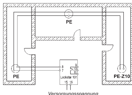
Prinzip-Anschluss mehrerer Plattenelektroden an ein Elektrodenrelais Leckstar 101 - Sammel- Alarmgabe
