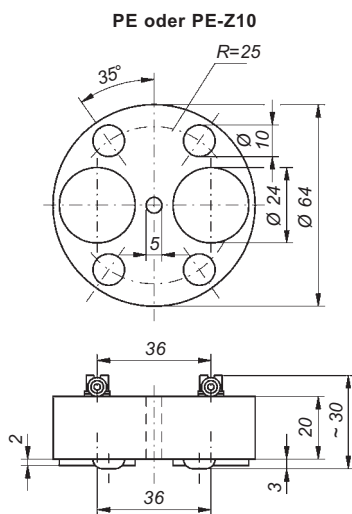
PE-Z10, Anschlussseite
