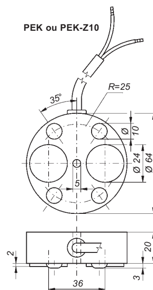
PEK-Z10, côté branchement
